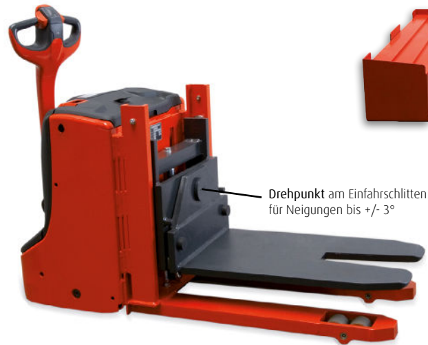
Gestufte Auflage für Batterien in den Größen 4, 5 und 6 PzS
